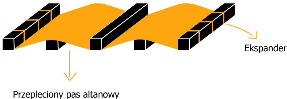
Rysunek 2. Proponowany sposób montażu pasów.
