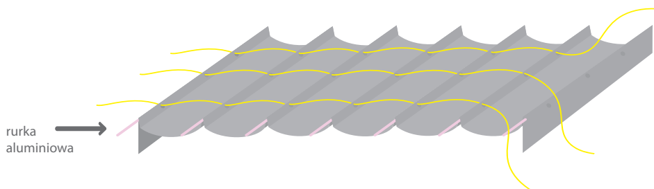
Rysunek 2. Montaż rolety rzymskiej
