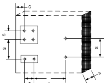
Schemat rozmieszczenia łączników w podłożu betonowym
