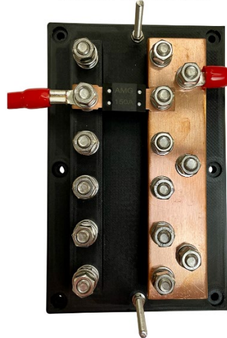
SZYNA DODATNIA
