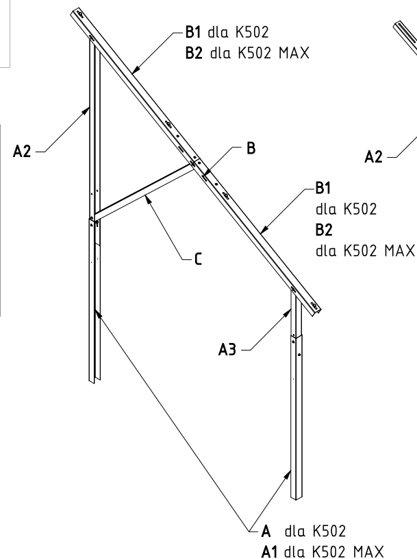
Rys.1a Kolumna podporowa (K502, K502 MAX)- Złożenie
