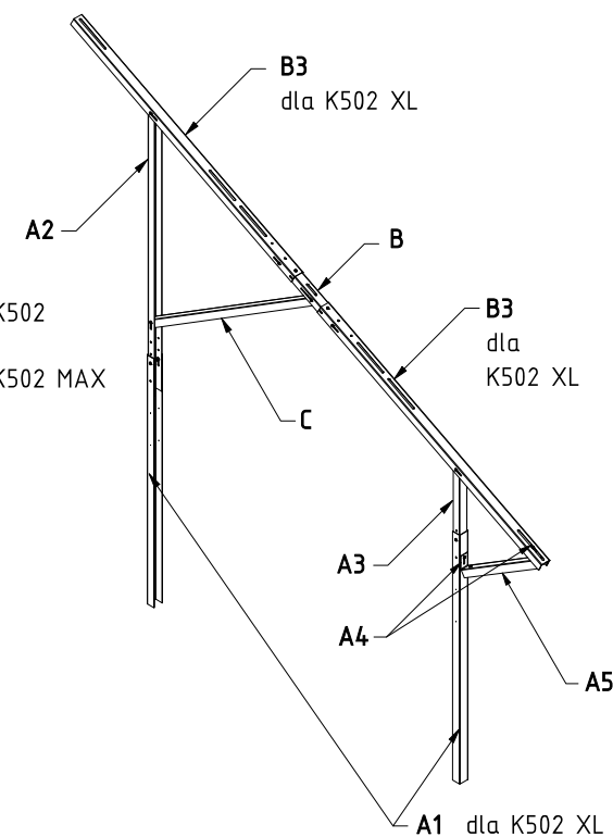
Rys.1b Kolumna podporowa (K502 XL)- Złożenie
