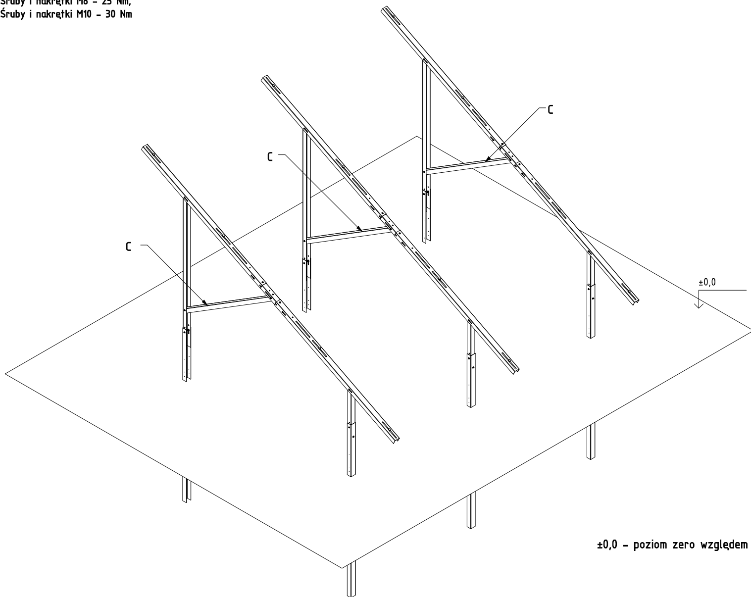
Rys.3-1 Złączenie zastrzału (C) z belką skośną
