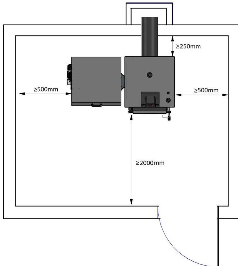
Rys. Usytuowanie kotła w kotłowni
