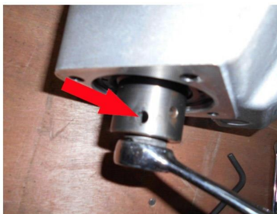
2. Kluczem ustawić trzpień ślimaka tak by było widać zerwaną śrubę
