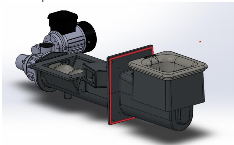
Rys. Przedstawia miejsce – flanszę mocującą do kotła gdzie należy uszczelnić palnik silikonem odpornym do 360stopni.
