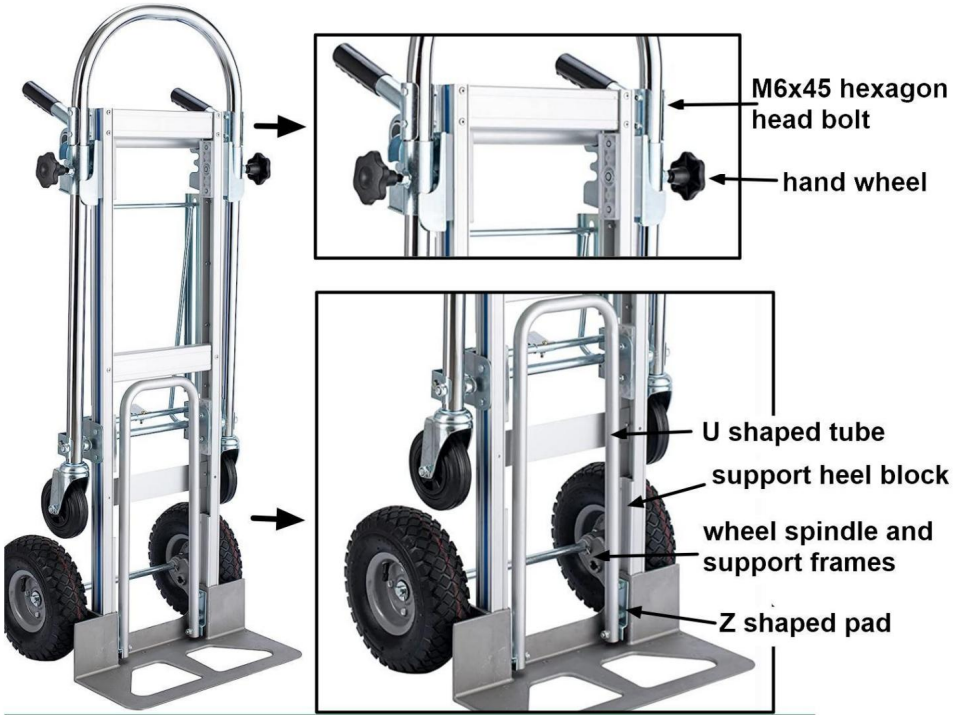
Fysiek detailldiagram
