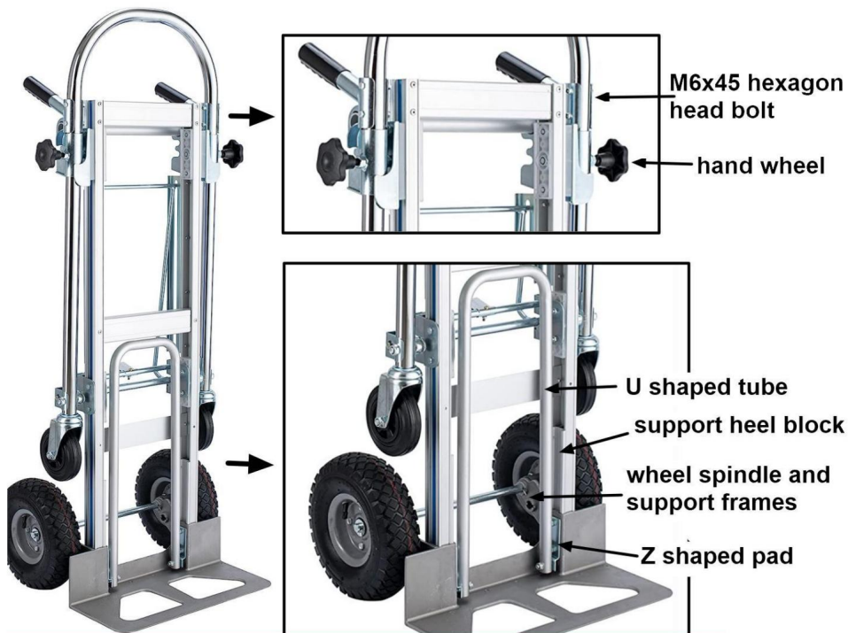
Fysiskt detaljdiagram
