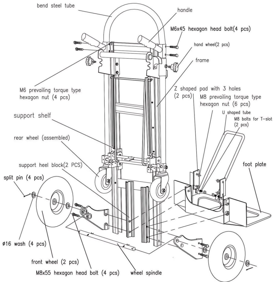
Anleitungsdiagramm
