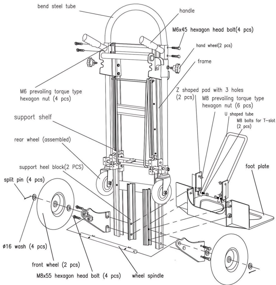
diagramme d'instructions
