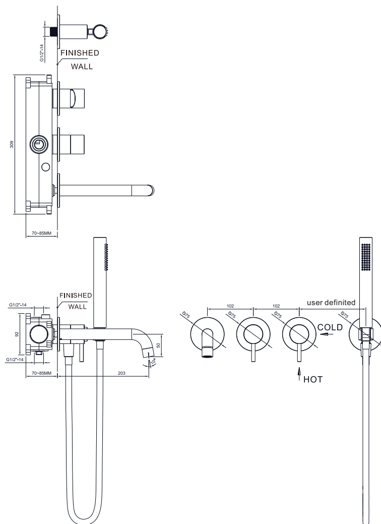
RYSUNEK TECHNICZNY
