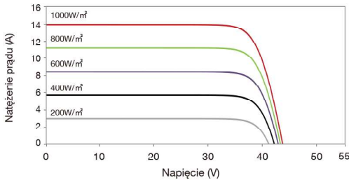
Wykres prądu w funkcji napięcia (60HL4-(V) 480W)
