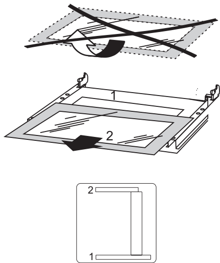
Wyjmowanie szyb wewnętrznych. 2 szyby.
