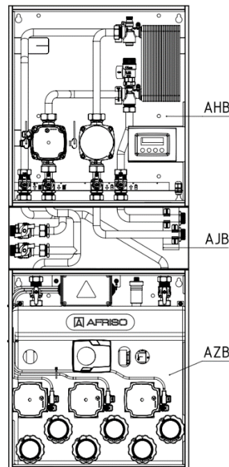
Rys. 5: Kolumna grzewcza AHB+AJB+AZB
