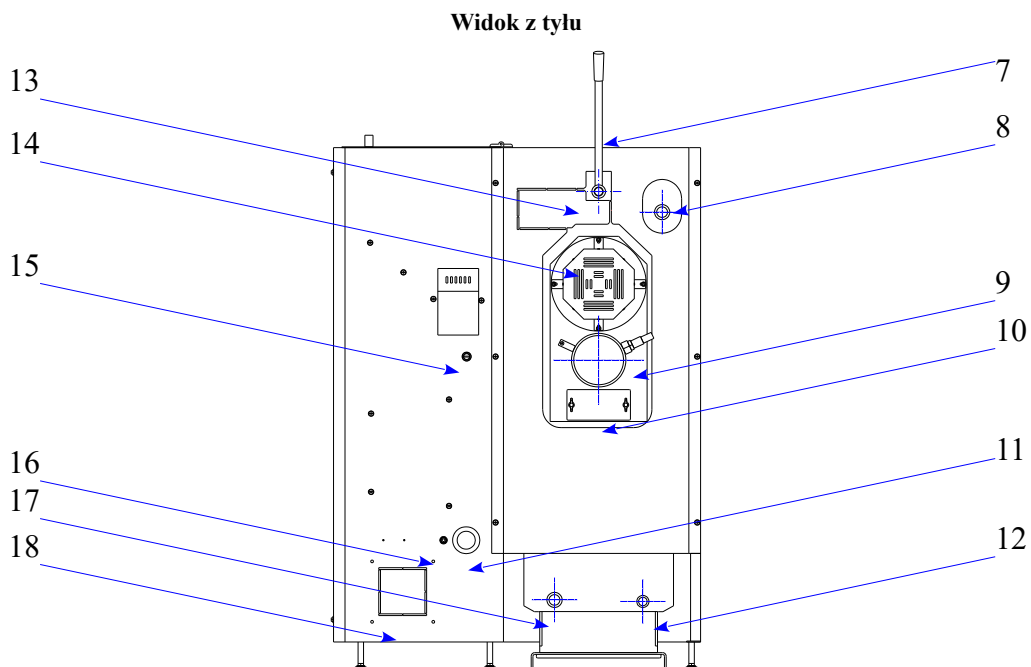
Rys nr 17. Opis schematyczny kotłów typu Smart Fire SF 11, SF15, SF15/3bar, SF22, SF22/3bar, SF31 oraz SF41: 7-dźwignia mechanizmu czyszczenia wymiennika; 8-króciec wody grzewczej; 9-czopuch spalinyowy wraz z czujnikiem temperatury spalin oraz sondą Lambda (wyposażenie opcjonalne); 10-wyczystka kolektora spalin; 11-przepust dla okablowania.; 12-króciec spustowy; 13-punkt montażu układu napędowego automatycznego systemu czyszczenia wymiennika (wyposażenie opcjonalne); 14-obudowa wentylatora wyciągowego; 15-reset termostatu bezpieczeństwa (pod plastikową nakrętką); 16-dławnica kabla zasilającego; 17-króciec wody powrotnej; 18-punkt montażu systemu zewnętrznej dystrybucji powietrza;
