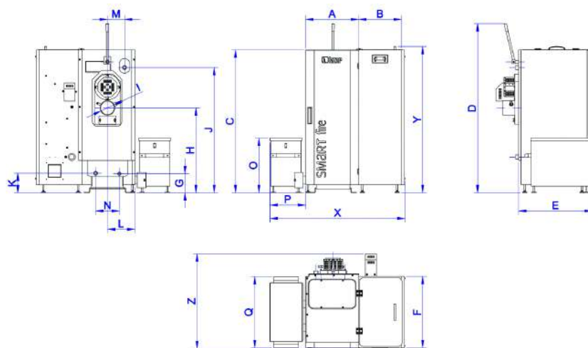
Rys nr 27. Wymiary kotłów Smart Fire SF11 COMPACT oraz SF15 COMPACT z systemem automatycznego odpowielania
