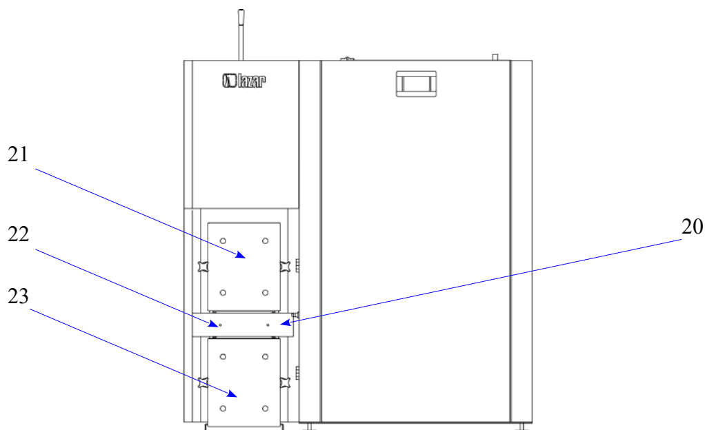
Rys nr 6. Opis schematyczny kotłów typu Smart Fire SF 11, SF15, SF15/3bar, SF22, SF22/3bar, SF31 oraz SF41 20-wyłącznik krańcowy maskownicy drzwi kotła; 21-drzwi komory palnika; 22-maskownica zapalarki ceramicznej oraz wyczystki palnika; 23-drzwi komory popielnika;
