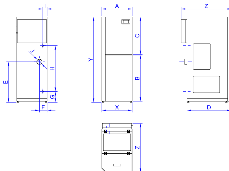
Rys nr 6. Opis schematyczny kotłów typu Smart Fire SF 11, SF15, SF15/3bar, SF22, SF22/3bar, SF31 oraz SF41 20-wyłącznik krańcowy maskownicy drzwi kotła; 21-drzwi komory palnika; 22-maskownica zapalarki ceramicznej oraz wyczystki palnika; 23-drzwi komory popielnika;
