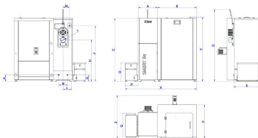
Rys nr 22. Wymiary kotłów Smart Fire SF11, SF15, SF15/3bar, SF22 oraz SF22/3bar z zasobnikiem paliwa 440L i systemem automatycznego odpowielania
