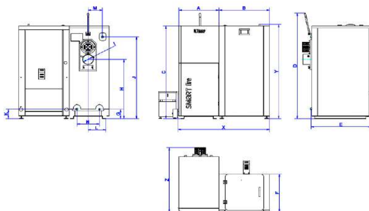
Rys nr 25. Wymiary kotłów Smart Fire SF31 oraz SF41 z zasobnikiem paliwa 240L i systemem automatycznego odpopielania
