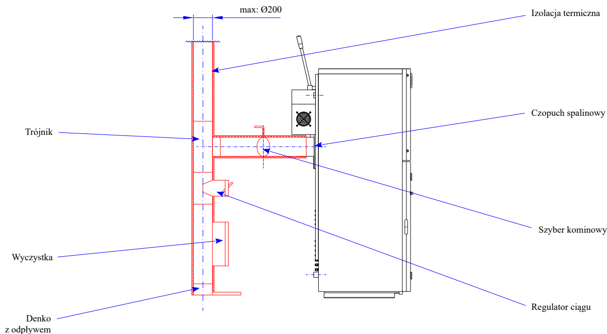
Rys nr 31. Przyłącze kominowe kotła Smart Fire
