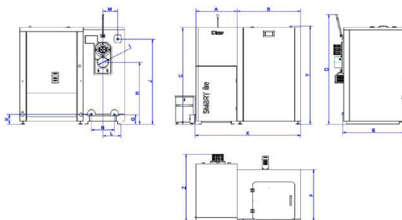
Rys nr 26. Wymiary kotłów Smart Fire SF31 oraz SF41 z zasobnikiem paliwa 440L i systemem automatycznego odpopielania
