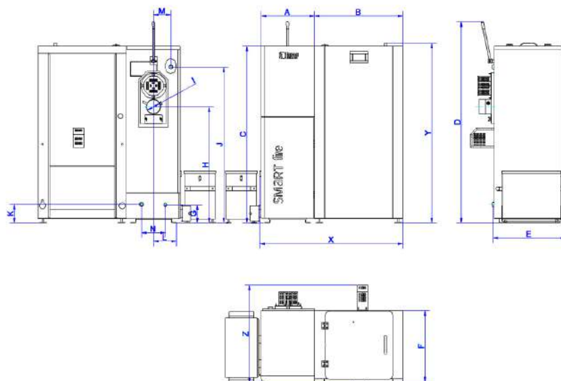
Rys nr 21. Wymiary kotłów Smart Fire SF11, SF15, SF15/3bar, SF22 oraz SF22/3bar z zasobnikiem paliwa 240L i systemem automatycznego odpowielania
