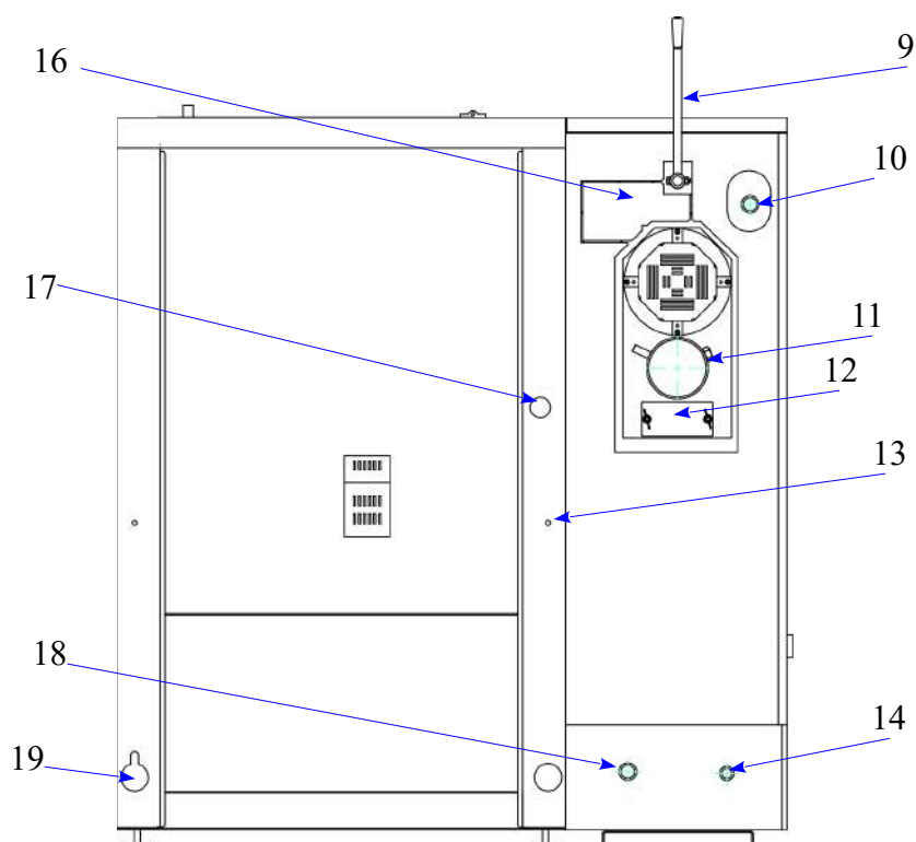
Rys nr 5. Opis schematyczny kotłów typu Smart Fire SF 11, SF15, SF15/3bar, SF22, SF22/3bar, SF31 oraz SF41: 9-dźwignia mechanizmu czyszczenia wymiennika; 10-króciec wody grzewczej; 11-czopuch spalinowy wraz z czujnikiem temperatury spalin oraz sondą Lambda (wyposażenie opcjonalne); 12-wyczystka kolektora spalin; 13-reset termostatu bezpieczeństwa STB (pod plastikową nakrętką); 14-króciec spustowy; 15-boczny panel rewizyjny; 16-punkt montażu układu napędowego automatycznego systemu czyszczenia wymiennika (wyposażenie opcjonalne); 17-przepust okablowania kolektora spalinowego; 18-króciec wody powrotnej; 19-dławnica kabla zasilającego wraz z przepustem dla okablowania;
