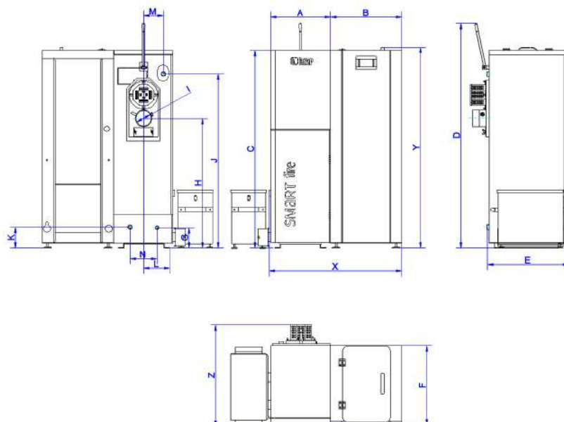
Rys nr 20. Wymiary kotłów Smart Fire SF11, SF15, SF15/3bar, SF22 oraz SF22/3bar z zasobnikiem paliwa 150L i systemem automatycznego odpopielania
