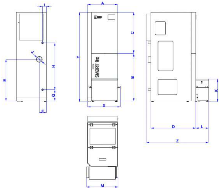
Rys nr 23. Wymiary kotła Smart Fire SF11 z zasobnikiem paliwa 130L i systemem automatycznego odpopielania
