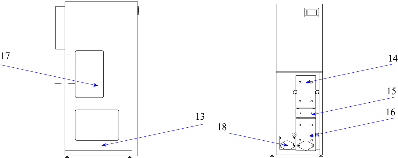
Rys nr 10. Opis schematyczny kotła Smart Fire SF11/130L 13-pokrywa otworu rewizyjnego; 14-drzwi komory spalania; 15-maskownica zapalarki ceramicznej oraz wyczystki palnika; 16-drzwi komory popielnika; 17-pokrywa otworu rewizyjnego czopucha spalinowego; 18-wyczystka dolnej części wymiennika ciepła;
