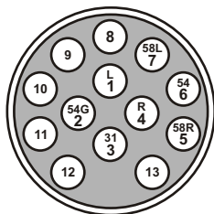
WIĄZKA DO PODŁĄCZENIA GNIĄZDA 13-BIEGUNOWEGO
