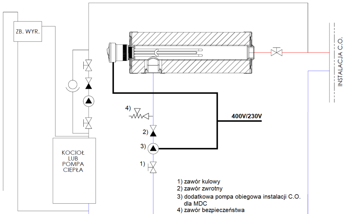
Rys. 3a. Przykładowy schemat montażu ogrzewacza typu MDC w instalacji C.O. systemu otwartego – pozioma pozycja instalacji.
