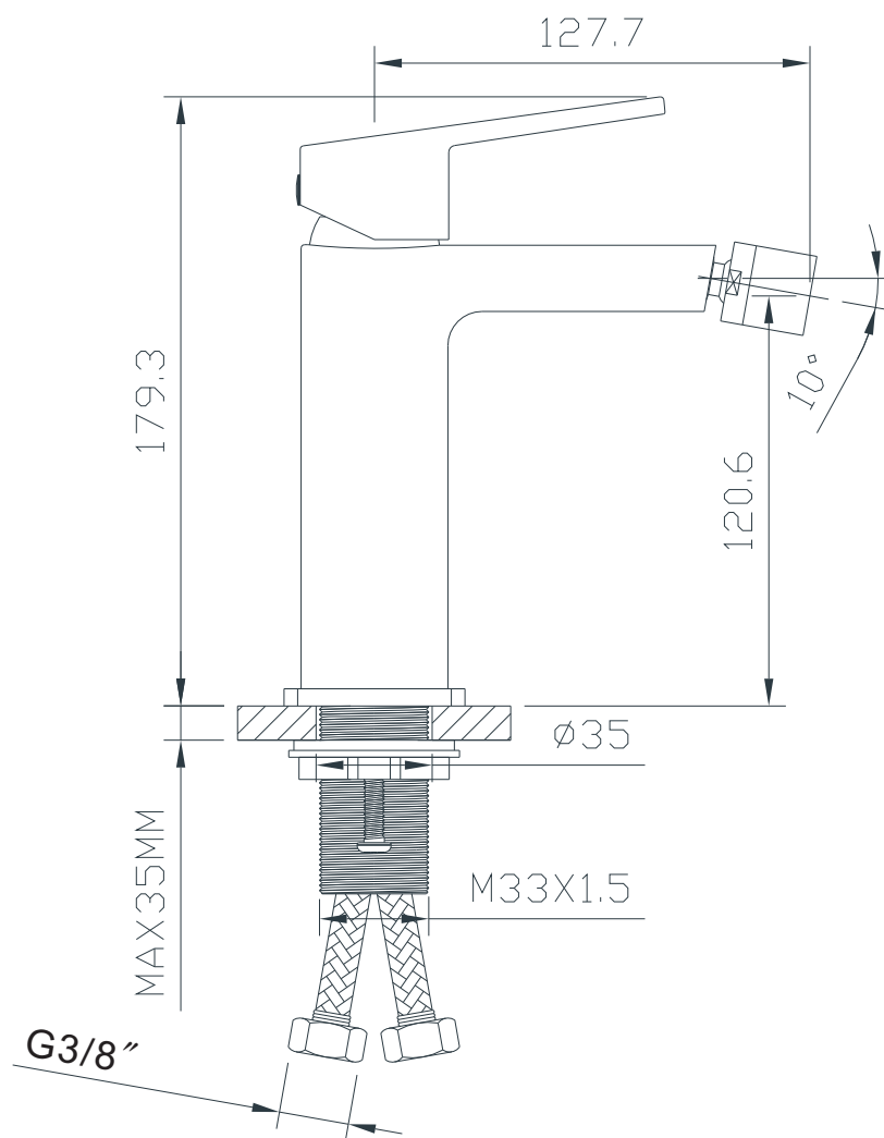
RYSUNEK TECHNICZNY
