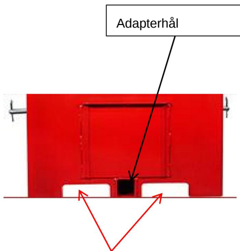
Gaffeltruck gränssnitt
