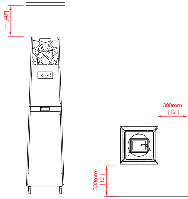
Rys. 2 – Odległości minimalne
