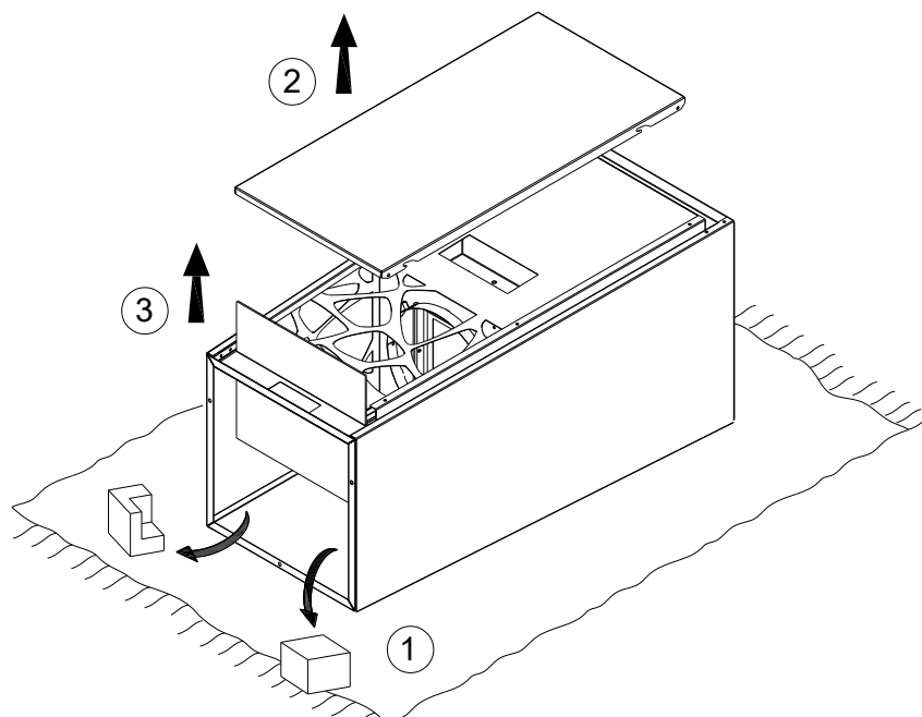
Rys. 4 – Rozpakowywanie kominka
