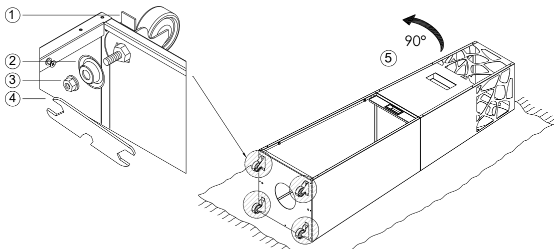
Rys. 7 – Montaż kół
