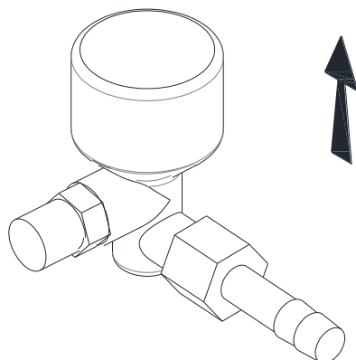
Rys. 10 – Zawór antyprzechyłowy
