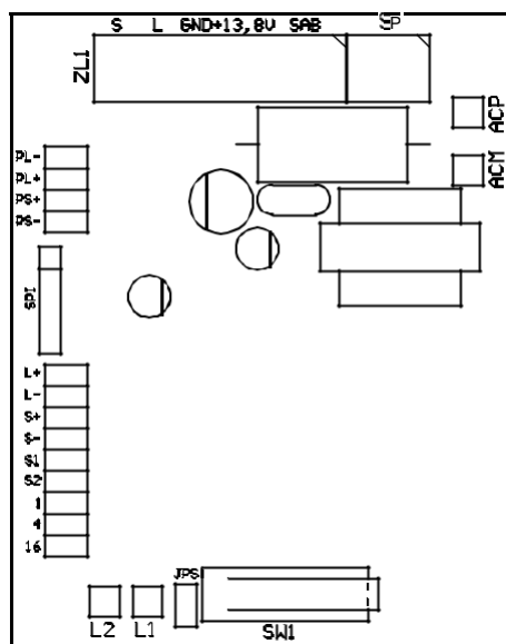
Rozmieszczenie wyprowadzeń i zwojów na płytce drukowanej
