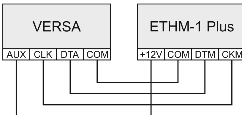
Rys. 6. Sposób podłączenia modułu ETHM-1 Plus do centrali.
