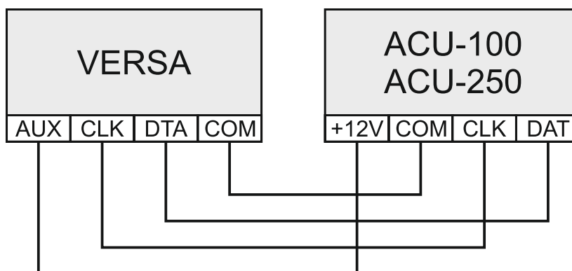
Rys. 12. Sposób podłączenia kontrolera ACU-100 / ACU-250 do centrali.
