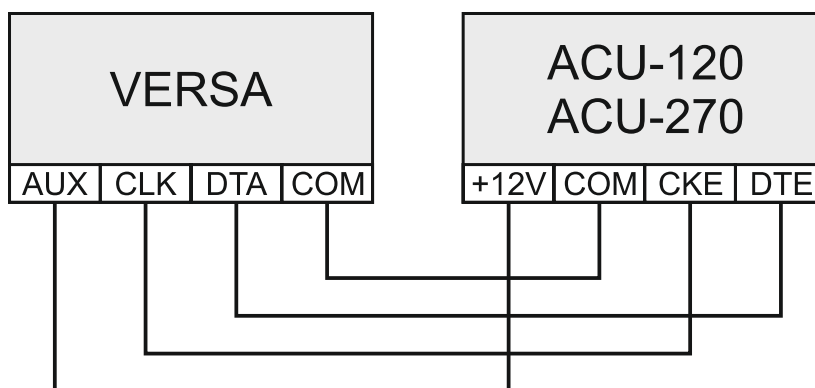
Rys. 11. Sposób podłączenia kontrolera ACU-120 / ACU-270 do centrali.
