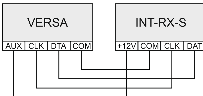
Rys. 8. Sposób podłączenia ekspandera INT-RX-S do centrali.
