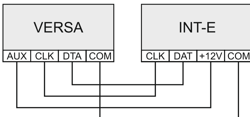
Rys. 15. Sposób podłączenia ekspandera INT-E do centrali.
