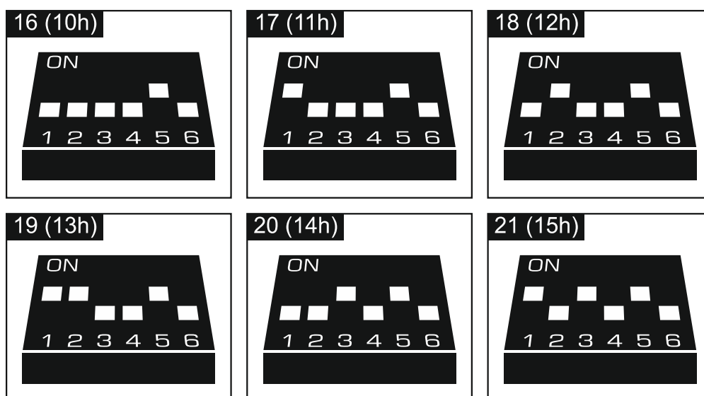
Rys. 20. Sposób ustawienia adresu na przykładzie modułu INT-IT / INT-IT-2.
