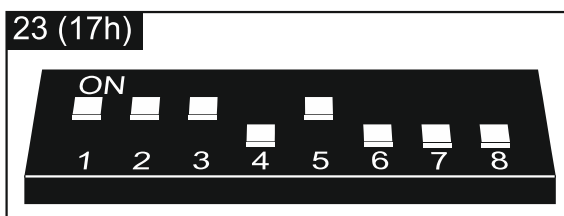
Rys. 21. Sposób ustawienia adresu w module INT-VG / ekspanderze CA-64 SM. Nagrywanie komunikatów głosowych jest zablokowane (przełącznik 8 w pozycji OFF).
