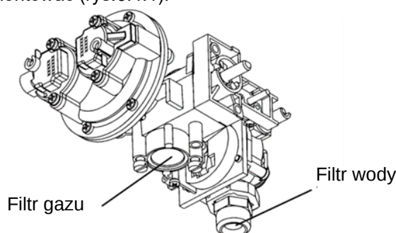
Rys 6.4.1. Armatura wodno-gazowa
