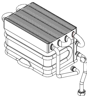
Rys. 6.1.1. Wymiennik ciepła
