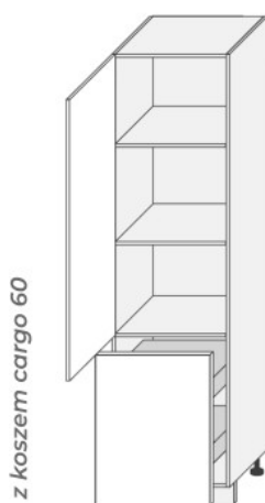
D14DP 60 (600/2070/565)
