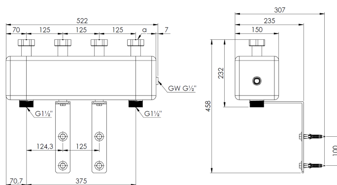
(a) - 4x nakrętka G1½"
