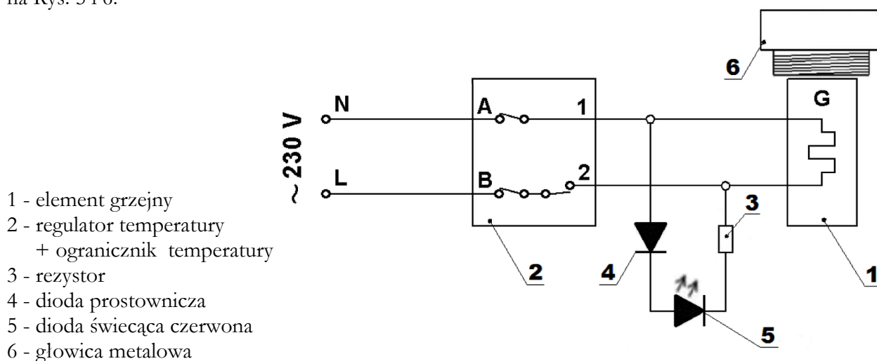
Rys. 5 Schemat elektryczny podgrzewacza z grzałką elektryczną 1- fazową
