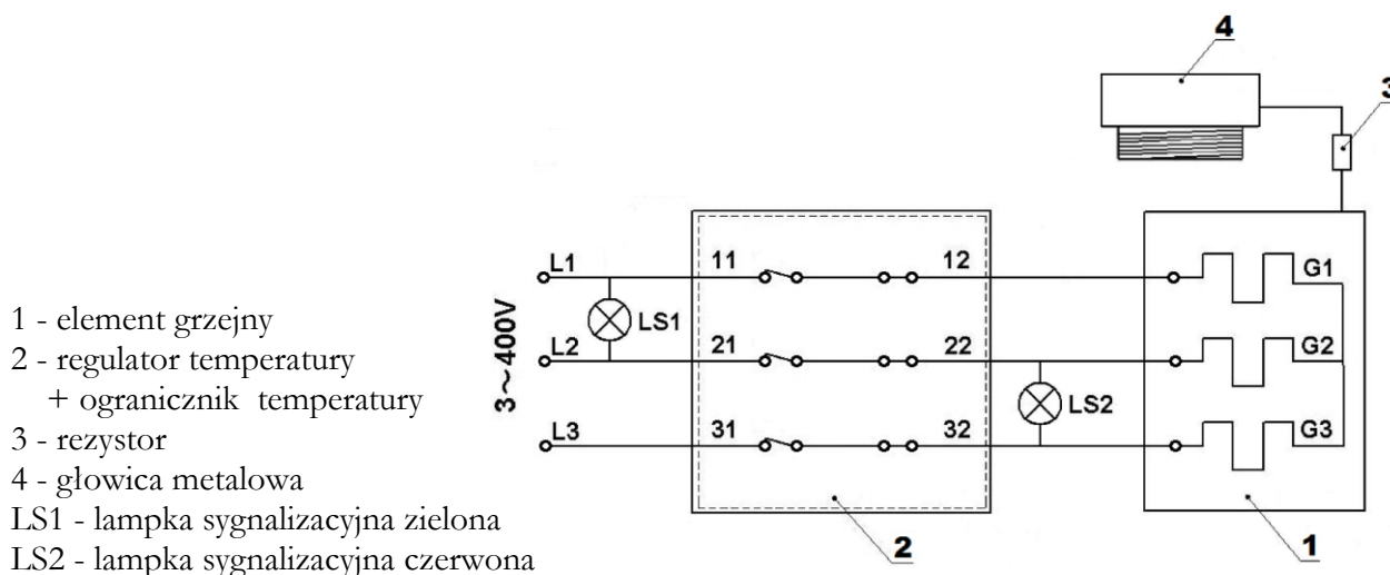
Rys. 6 Schemat elektryczny podgrzewacza z grzałką elektryczną 3- fazową
