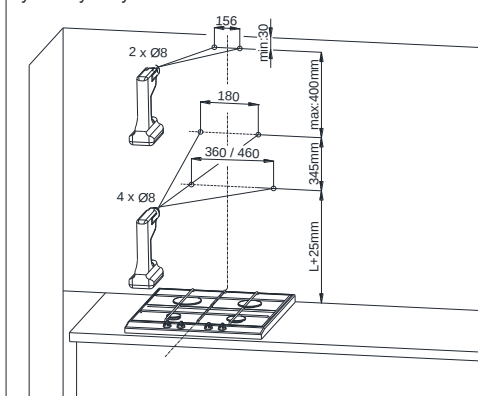
Rys. 6 Zawieszanie okapu.
