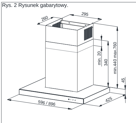
Rys. 2 Rysunek gabarytowy.
