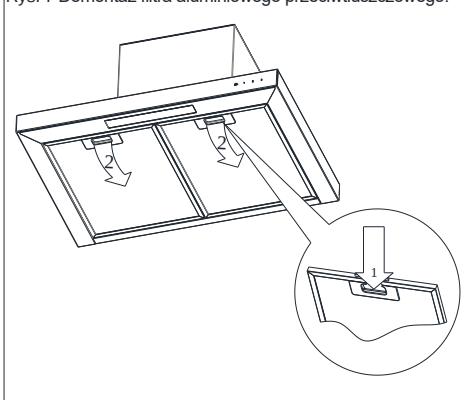
Rys. 7 Demontaż filtra aluminiowego przeciw tłuszczowego.
