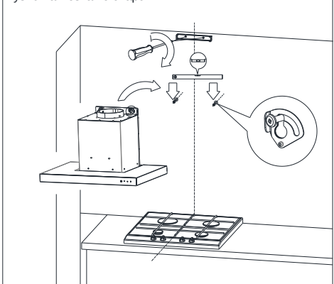
Rys. 6 Zawieszanie okapu.
