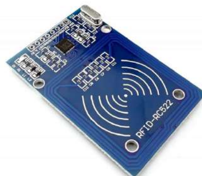
Moduł czytnika RFID RC522
