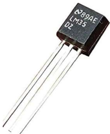
LM35DZ analogow czujnik temperatury
