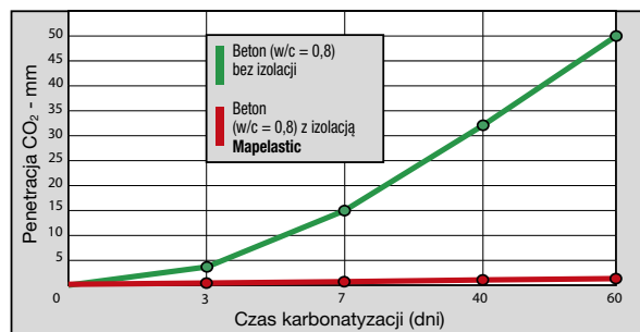
Rys. 2 Wpływ izolacji Mapelastic na ograniczenie karbonatyzacji (30% CO 2 ) w betonie.
