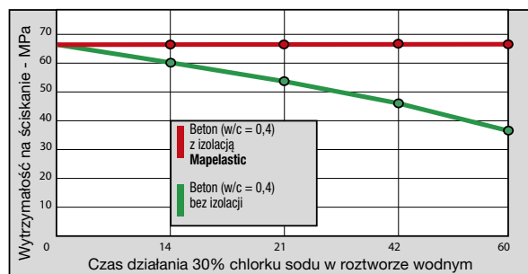
Rys. 4 Wpływ izolacji Mapelastic na ograniczenie spadku wytrzymałości betonu spowodowanego działaniem soli odładowych, zawierających chlorek wapnia.
