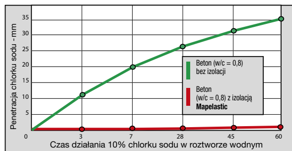
Rys. 3 Wpływ izolacji Mapelastic na ograniczenie penetracji chlorków sodu w porowatym betonie.
