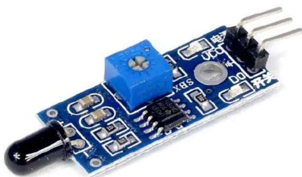
Czujnik płomieni
