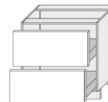
D2A 80 (800/820/500)
