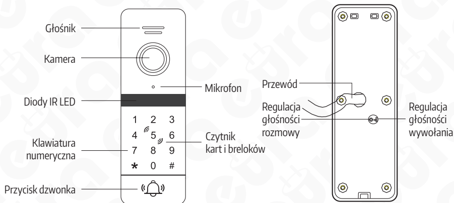
Rys. 1 Budowa kasey zewnętrznej
