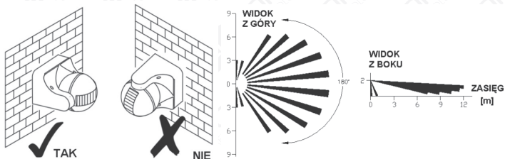
Rys. 4. Przykład prawidłowego i nieprawidłowego montażu czujnika
