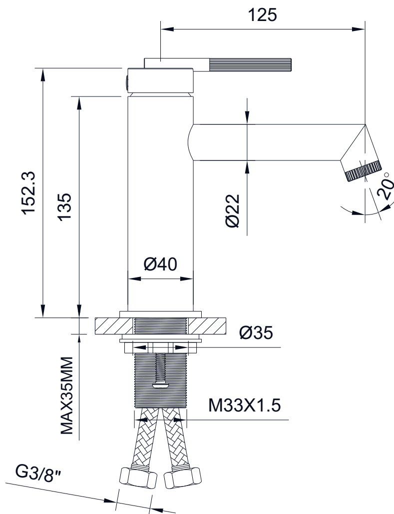
RYSUNEK TECHNICZNY
