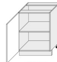
D1D 60 (600/820/500)
