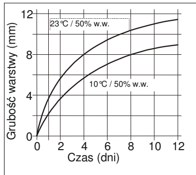
Wyk. 1.: Szybkość utwardzania Sikaflex 221
