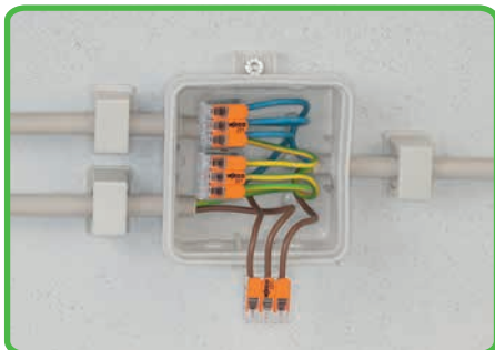
Oprzewodowanie puszkii instalacyjnej przy użyciu przewodów linkowych
