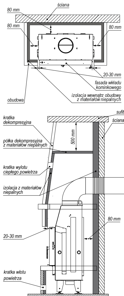
Rysunek 6. Przykładowa zabudowa wkładu kominkowego.
