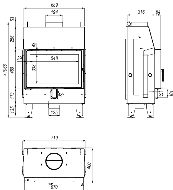
Rysunek 2. Wymiary wkładu kominkowego IMPULS SM.
