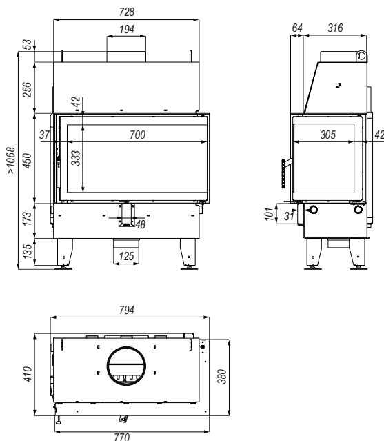
Rysunek 5. Wymiary wkładu kominkowego IMPULS ME w wersji BP i BL (odbicie lustrzane wersji BP).
