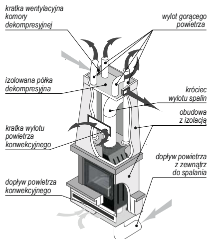
Rysunek 7. System dystrybucji gorącego powietrza.
