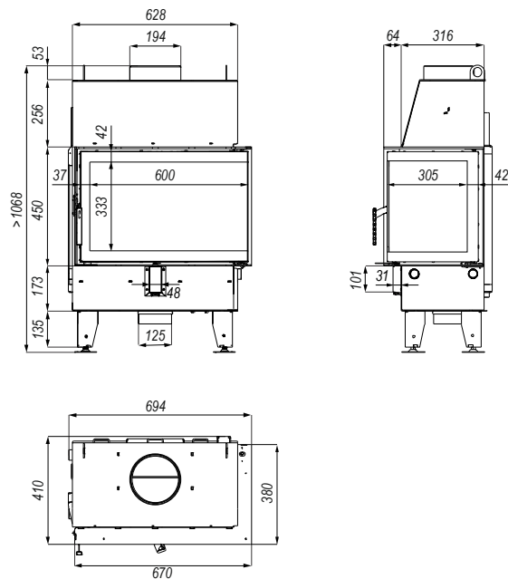
Rysunek 4. Wymiary wkładu kominkowego IMPULS SM w wersji BP i BL (odbicie lustrzane wersji BP).
