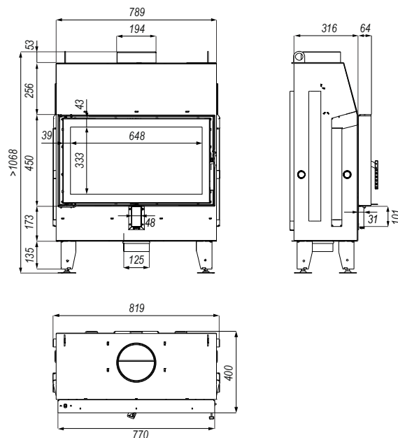
Rysunek 3. Wymiary wkładu kominkowego IMPULS ME.
