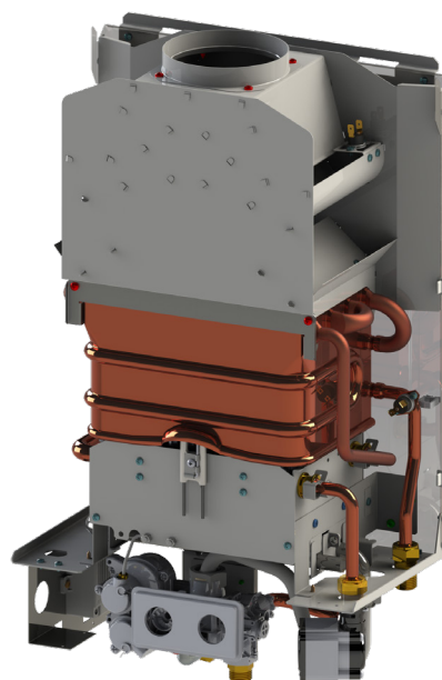
TERMAQ AQUA POWER ECO zapłon elektroniczny z hydrogeneratora
