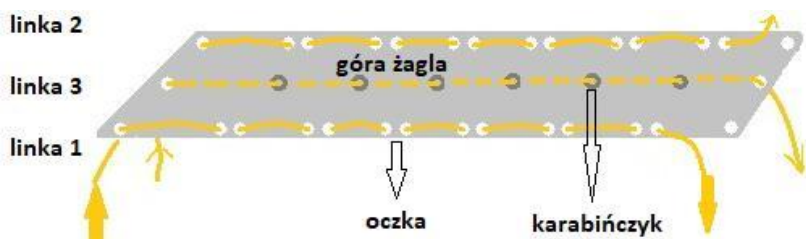
Rysunek 2. Proponowany sposób montażu żagla (trzecia linka jest opcjonalna).
