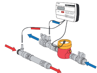
Przykład montażu przetwornika przepływu na powrocie
