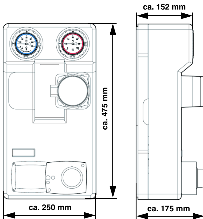
Abbildung 3: PrimoTherm® Standardausführung
