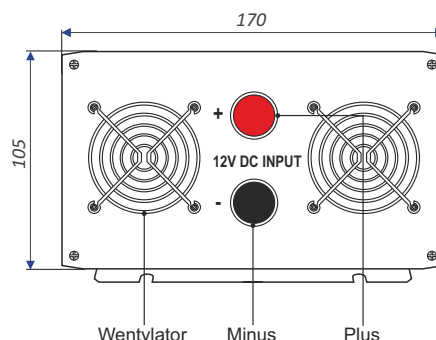
Panel wejściowy akumulatora DC
