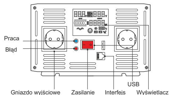
Panel wyjściowe AC
