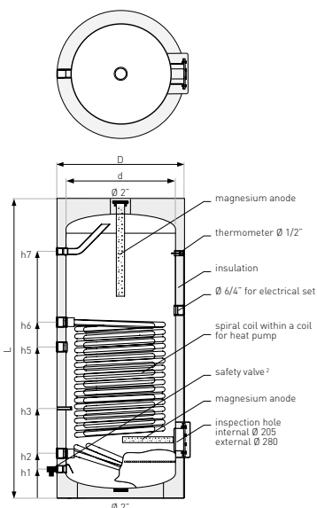
scheme - SGW(S) Maxi 700-1500
