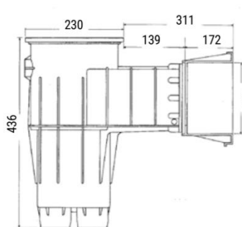
Skimmer z dużym otworem - 3119
