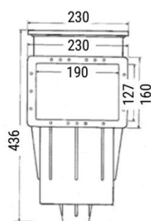
Skimmer z małym otworem - 3111
