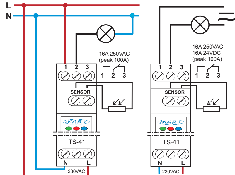
Rys. 2.: Schematy podłączenia AUTOMATU ZMIERZCHOWEGO TS-41-3.4.
