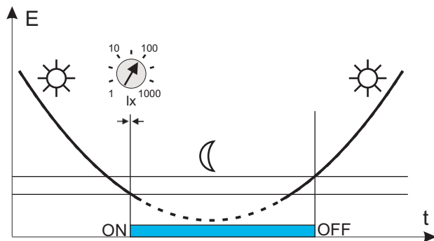
Rys. 3.: Schematy poglądowy zasady działania AUTOMATU ZMIERZCHOWEGO TS-41-3.4
