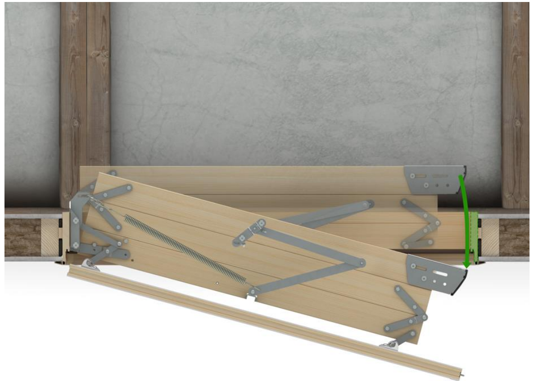
Rys.2 Odległość zamachowa schodów ze stopkami LXS-W
