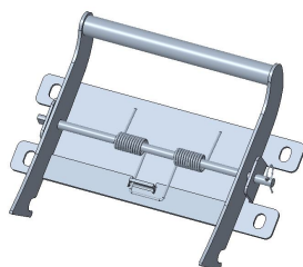
Cadre de verrouillage (x1)
