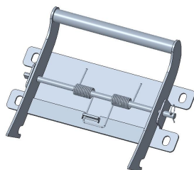
Rama blokująca (x1)
