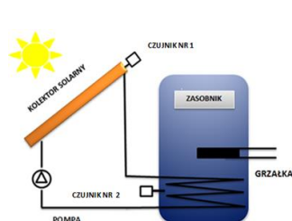
2. Ładowanie zasobnika C.W.U z funkcją dogrzewania grzałką, konieczne rozbudowanie o część wykonawczą (stycznik)
