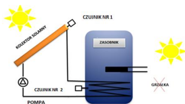
4. Ładowanie zasobnika C.W.U z funkcją dogrzewania grzałką, a priorytetem dla dogrzewania przez kolektor. Ogranicza zużycie energii elektrycznej. Konieczne rozbudowanie o część wykonawczą- stycznik.
