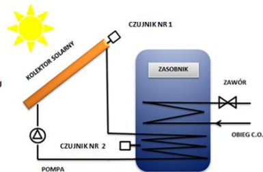
3. Ładowanie zasobnika C.W.U przez kolektor solarny oraz kocioł C.O dwie węzłownice
