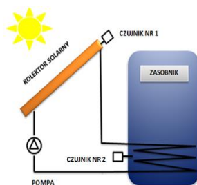
1. Ładowanie zasobnika C.W.U przez kolektor solarny. (Wersja podstawowa)
