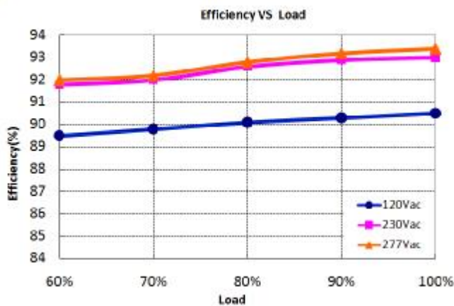
X6-200Y191 (Io=1.05A)
