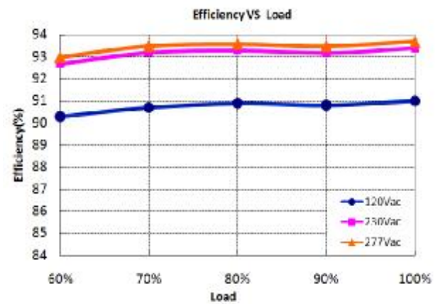
X6-200Y191 (Io=1.50A)
