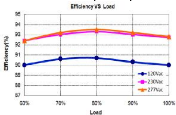
X6-200Y143 (Io=1.40A)
