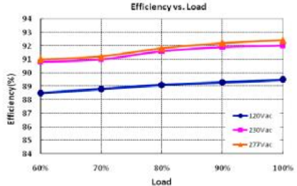
X6-200Y286 (Io=1.05A)
