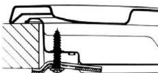
Położenie haka H=30mm od góry
