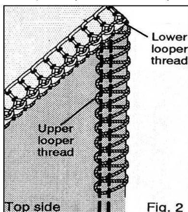
Увеличить натяжение нити верхнего петлителя и / или уменьшить натяжение нижнего
