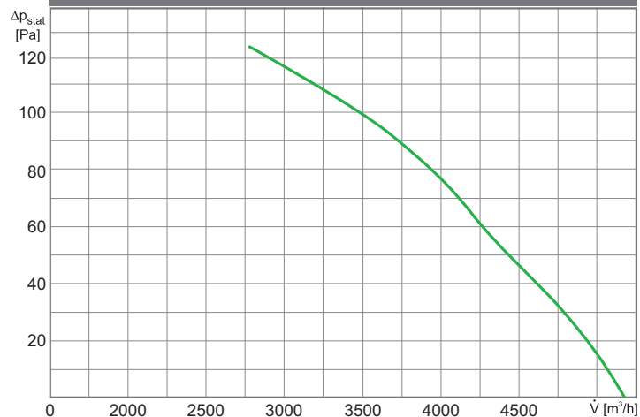
WAX 450/W/4/5100S
