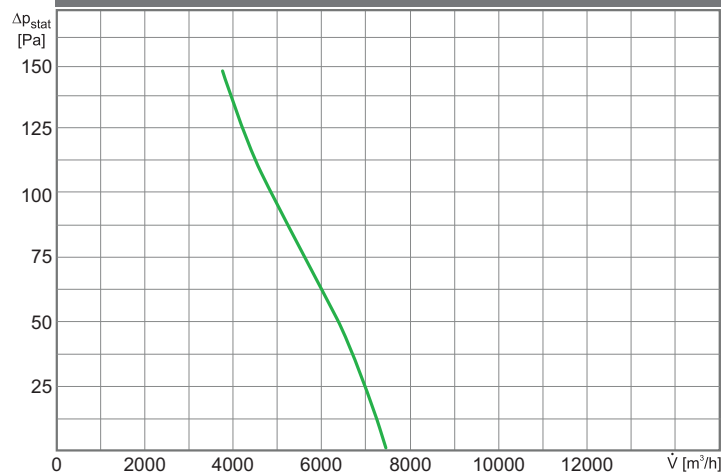
WAX 550/W/4/7500S
