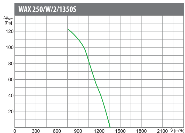
charakterystyki pracy
